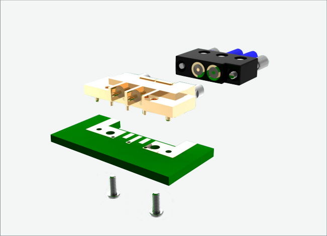
Edge Mount
